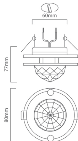
D103 CAD DIAGRAM
