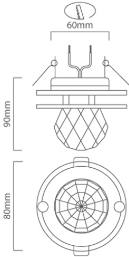
D104 CAD DIAGRAM
