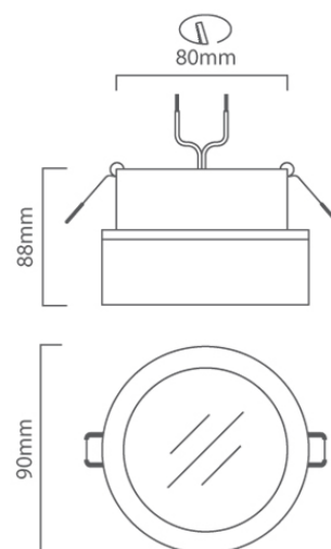
D105 CAD DIAGRAM
