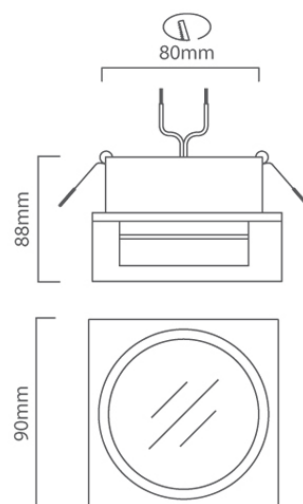
D106 CAD DIAGRAM
