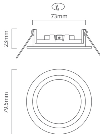
D108 CAD DIAGRAM
