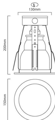
D10 CAD DIAGRAM
