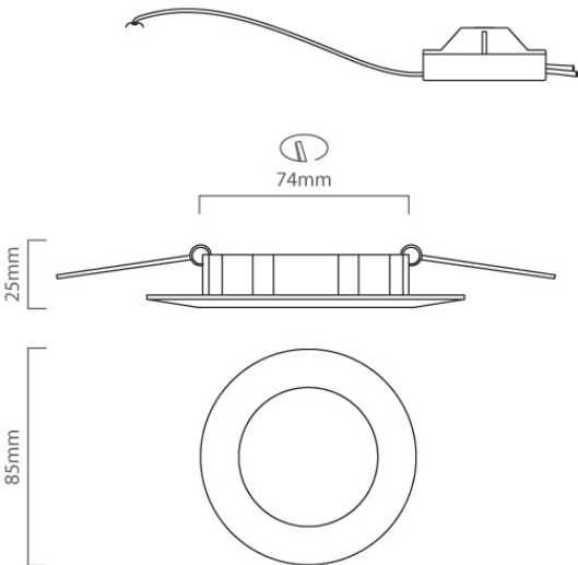
D110 CAD DIAGRAM
