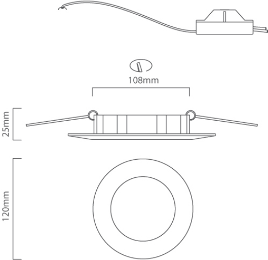
D112 CAD DIAGRAM
