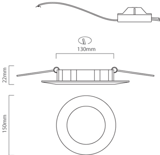
D113 CAD DIAGRAM
