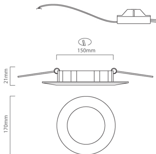
D114 CAD DIAGRAM
