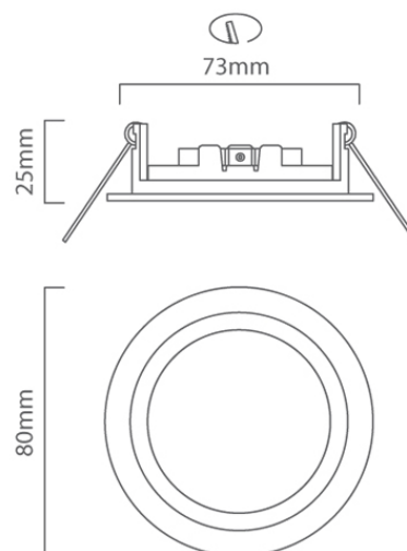
D18 CAD DIAGRAM
