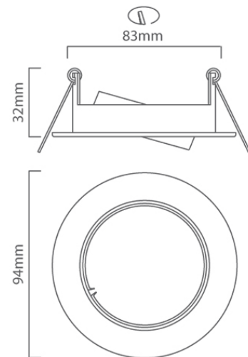
D19 CAD DIAGRAM
