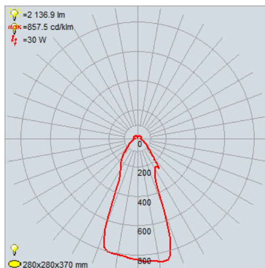
D25 IES DIAGRAM
