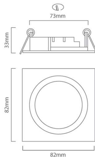
D56 CAD DIAGRAM
