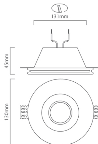
D94 CAD DIAGRAM
