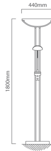
FL90 CAD DIAGRAM
