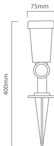
O113 CAD DIAGRAM
