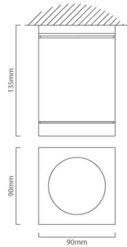
O135 CAD DIAGRAM
