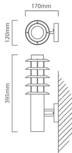
O143 CAD DIAGRAM
