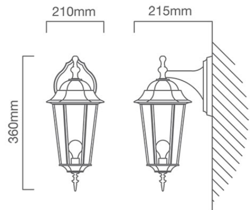
O18 CAD DIAGRAM
