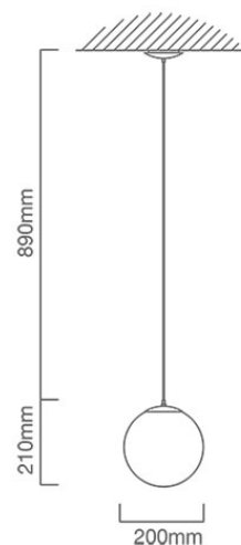
P198 CAD DIAGRAM
