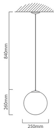
P199 CAD DIAGRAM
