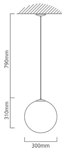
P200 CAD DIAGRAM
