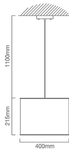
P363 CAD DIAGRAM
