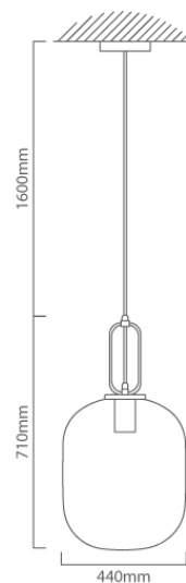
P901CL CAD DIAGRAM
