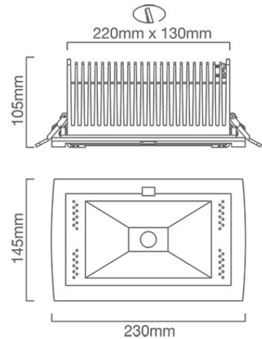
PR343 CAD DIAGRAM
