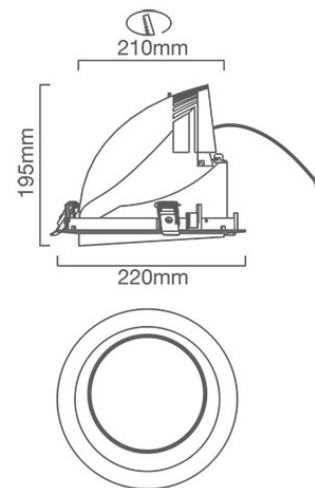
PR344 CAD DIAGRAM
