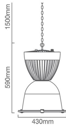
PR361 CAD DIAGRAM
