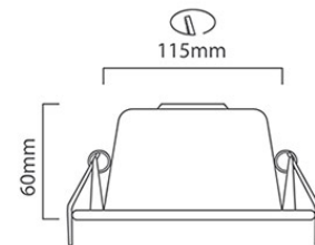
PR457 CAD DIAGRAM
